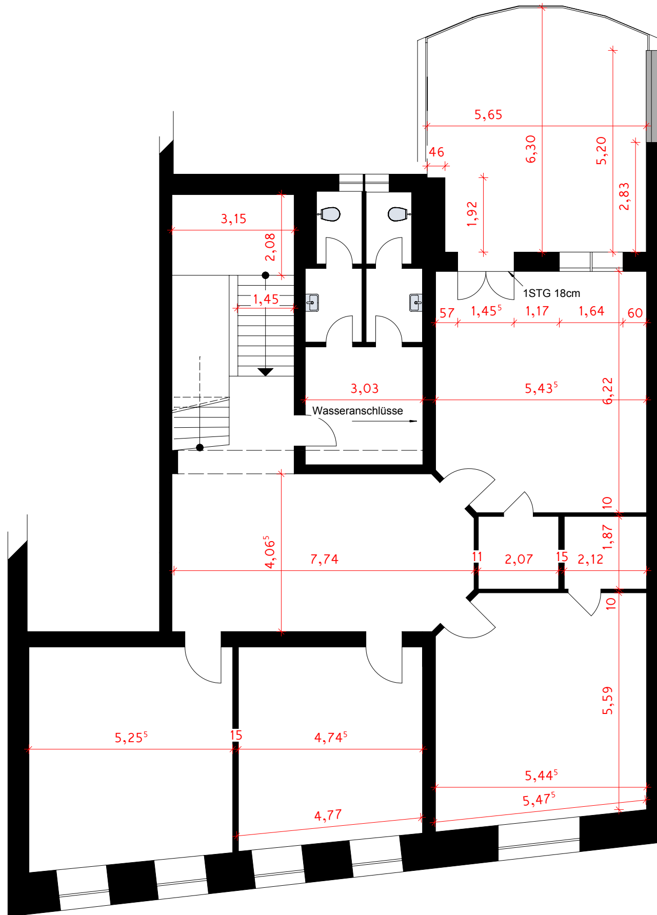
Teilbereich 1.Obergeschoss
